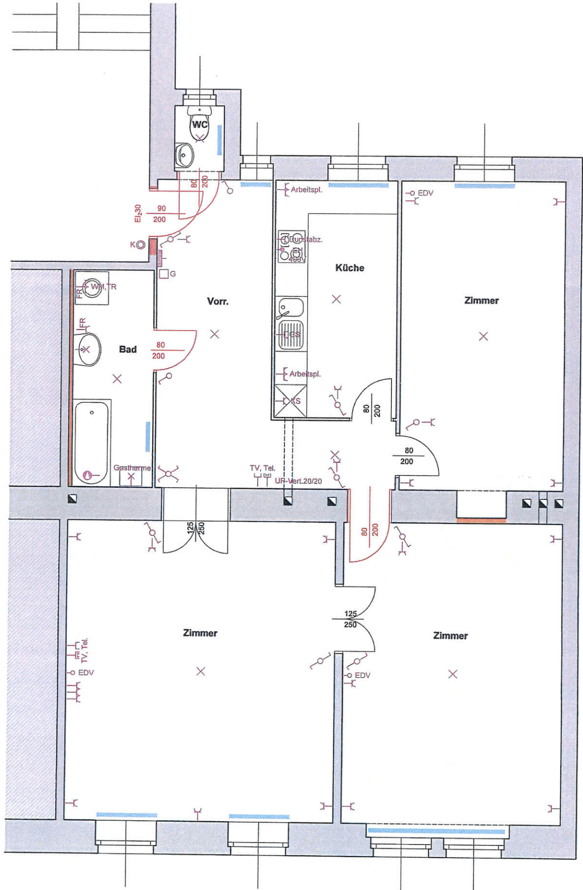
GRUNDRISS 1.Obergeschoss
